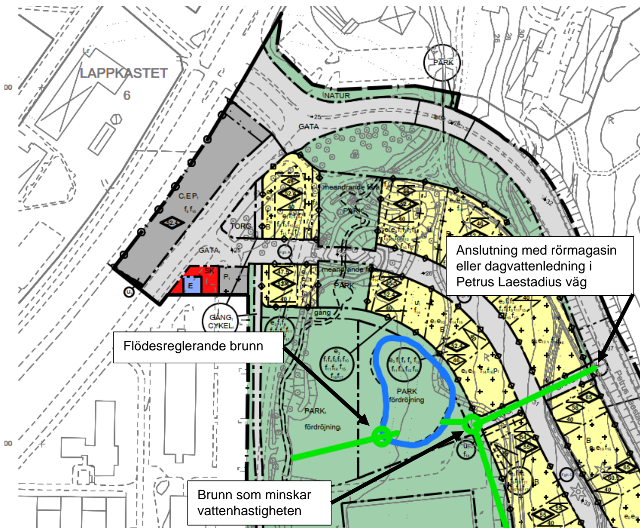
Figur 11. Principskiss för dagvattenmagasinet Bönan.
