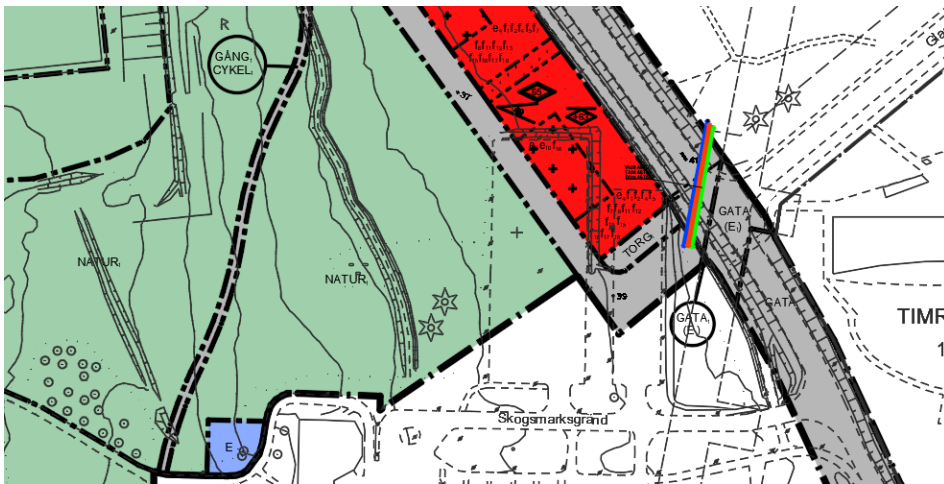
Figur 10. Ledningskorsningar i Petrus Laestadius väg utan anslutning mot U-område.
