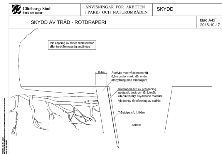
Exempel på typritning av rotdraperi
