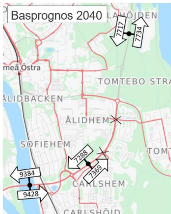
Figur 3-2 Trafikflöden (ÅDT) på Östra länken (E4) enligt basprognos 2040. Kryssade cirkulationsplatser visar att de inte är modellerade i Sampers. Baskarta från OpenStreetMap.
