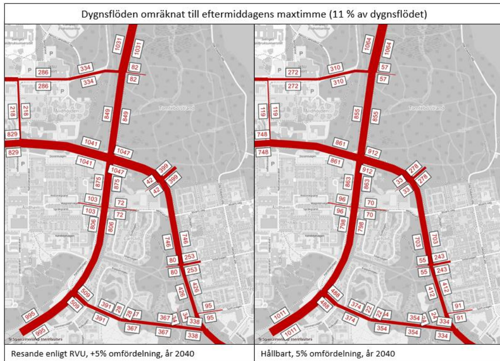
Figur 4-1 Trafikflöden under eftermiddagens maxtimme, kl 16-17. Samtliga resrelationer i Visum-matrisen har räknats ner till 11 %.
